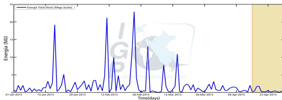
Figura 3.- Evolución de la Energía sísmica total diaria asociada a la actividad del volcán Misti entre los días 01 de Enero y el 30 Abril 2015. El área sombreada corresponde al periodo del presente reporte.
