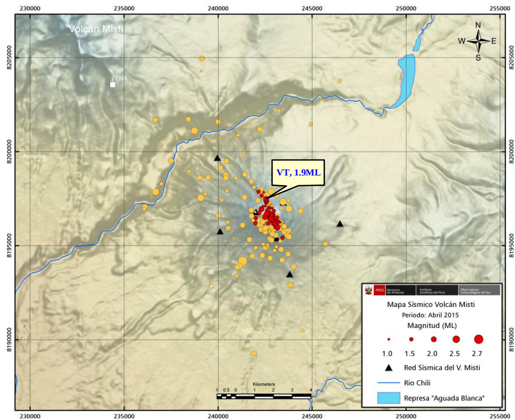
Figura 1.- Distribución epicentral de sismos de tipo fractura (VT), registrados en Abril 2015 (círculos rojos). El evento de fractura más energético en la última quincena, fue el sismo del 18 de Abril a las 11:05 Hora Local de 1.9ML, localizado a 1 km del cráter en el flanco Nor-Oeste del volcán. Los círculos en amarillo corresponden a sismos ocurridos entre Enero y Marzo 2015.
