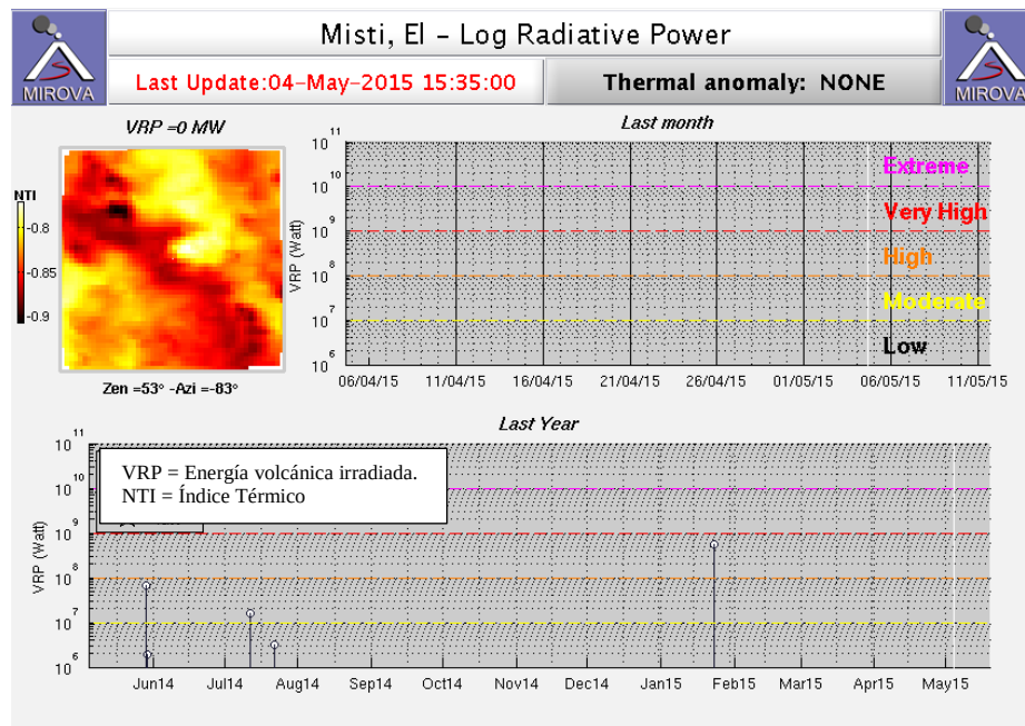
Figura 4.- Monitoreo térmico satelital en tiempo cuasi-real MIROVA: en este periodo 16-30 Abril no hay ninguna anomalía térmica asociada al volcán Misti.
