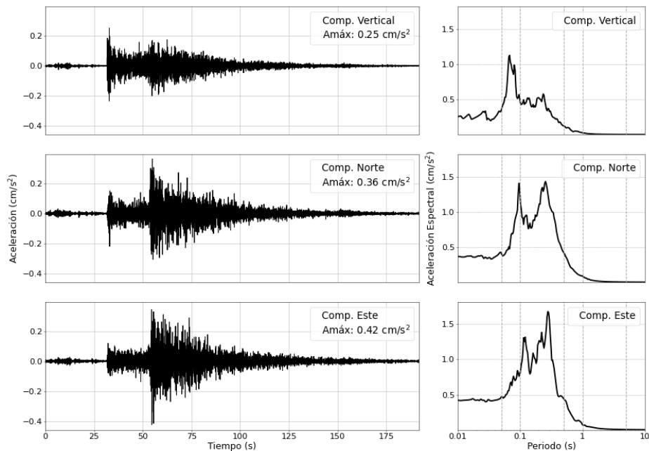
Figura 3: Registros de aceleración para el sismo del 27/07/2026 (M4.6) y sus correspondientes espectros de respuestas con amortiguamiento al 5 %
