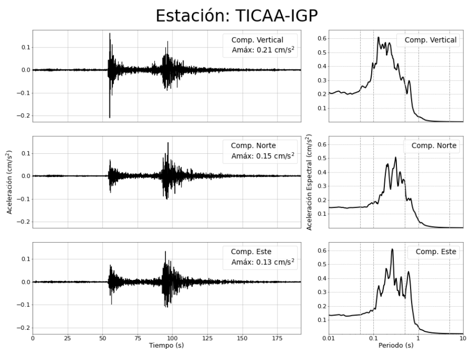
Figura 7: Registro de aceleración para el sismo del 27/07/2026 (M4.6) y sus correspondientes espectros de respuestas con amortiguamiento al 5 %
