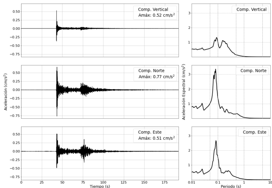
Figura 5: Registros de aceleración para el sismo del 27/07/2026 (M4.6) y sus correspondientes espectros de respuestas con amortiguamiento al 5 %
