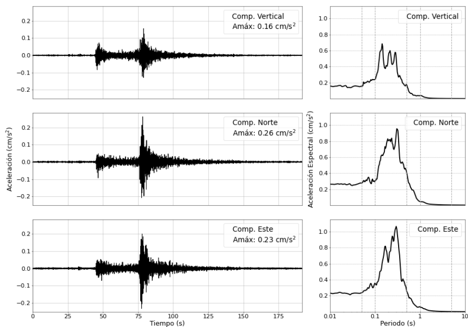
Figura 6: Registros de aceleración para el sismo del 27/07/2026 (M4.6) y sus correspondientes espectros de respuestas con amortiguamiento al 5 %
